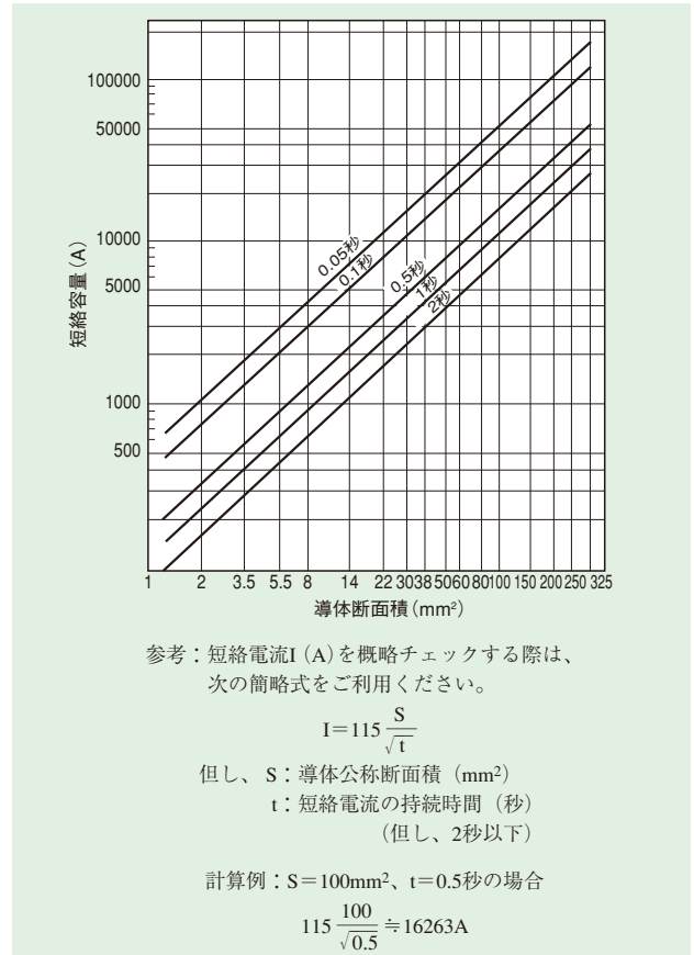
図2. MLFCの短絡容量
