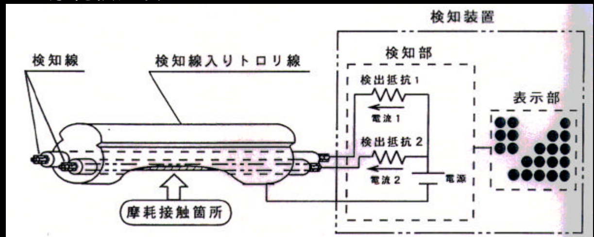
トロリ線摩耗検知原理
